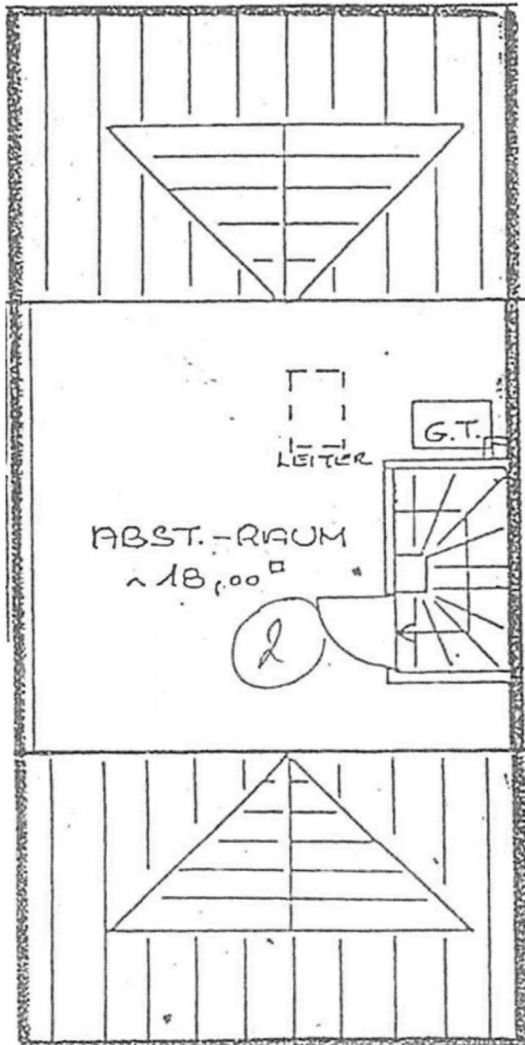
Grundriss Dachgeschoss
