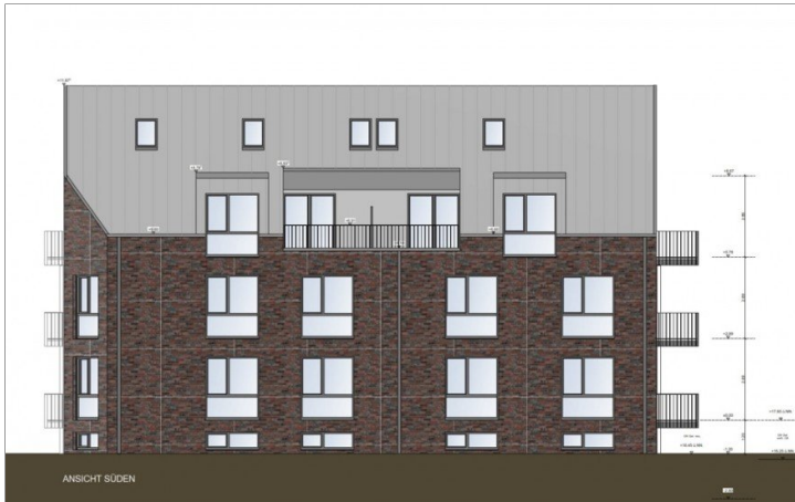
ANSICHT SÜDEN
