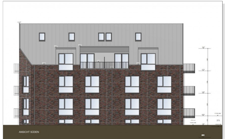
ANSICHT SÜDEN
