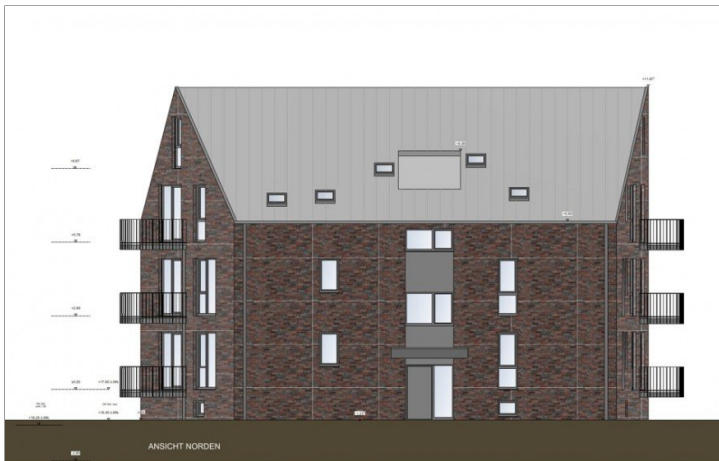
ANSICHT NORDEN
