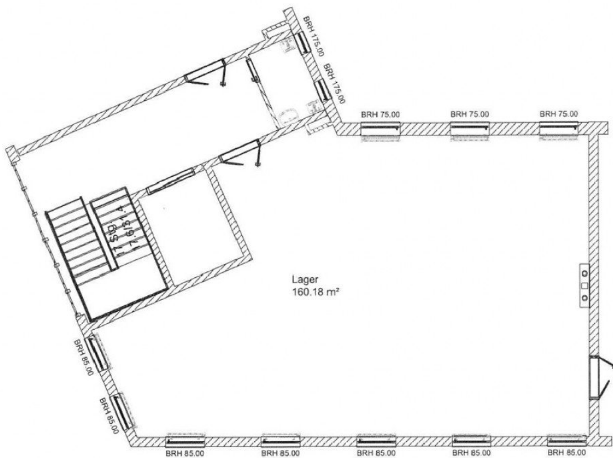
Grundriss Lagerfläche
